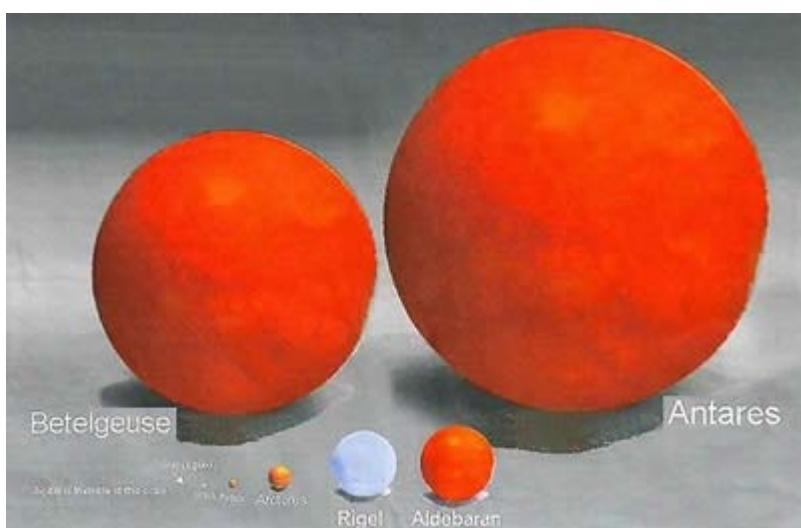
Изображение 4: Посмотрите на звезду Арктурус в сравнении со звездой Антарес. Даже планета Юпитер («твой» Гуру) уже не видна теперь. «Твое» солнце, – Бог, – всего лишь точка, которую можно рассмотреть только под микроскопом. А это звезда Антарес – 15-ая звезда. Есть еще 14 звезд кроме Антареса, они еще больше, намного больше!
