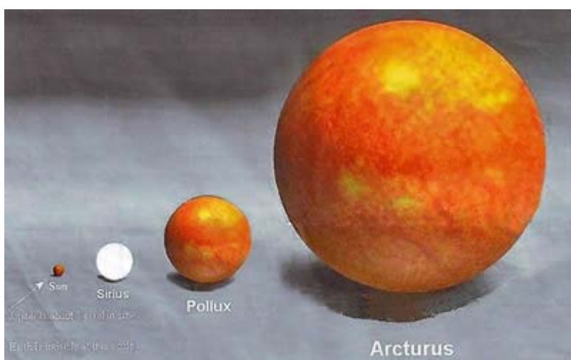
Изображение 3: Посмотрите на звезду Солнце в сравнении со звездой Арктурус. Земля уже не видна.
